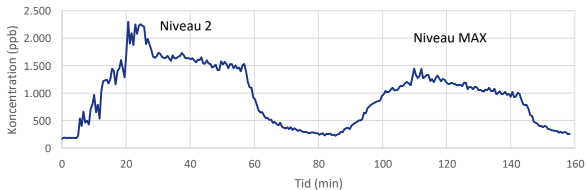
Figur 7. TVOC-koncentration for AeroGuard 4S med forfilter på niveau 2 og MAX.
