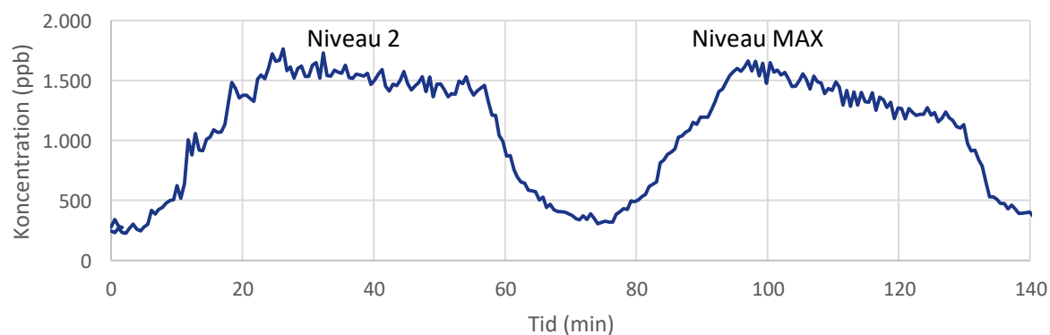
Figur 4. TVOC-konzentration for AeroGuard 4S på niveau 2 og MAX.
