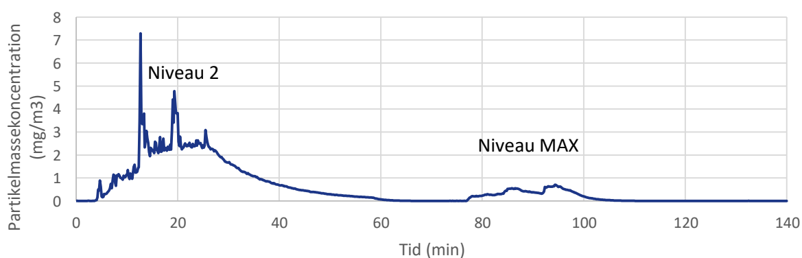
Figur 3. Total partikelmassekonzentration for AeroGuard 4S på niveau 2 og MAX.
